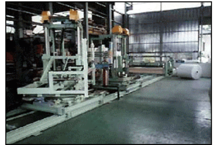
自動機・養生打自動添付装置 SS400製 設計・製作・据付
